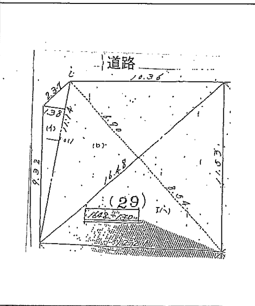
測量図 (1/250を50%縮小)
