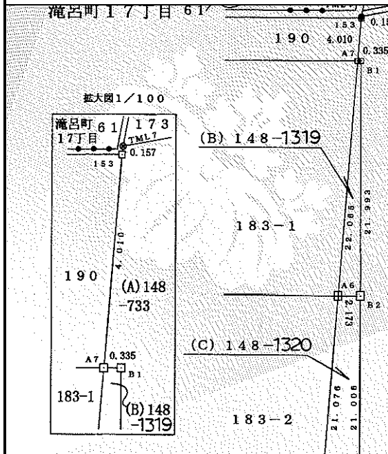
求積図
