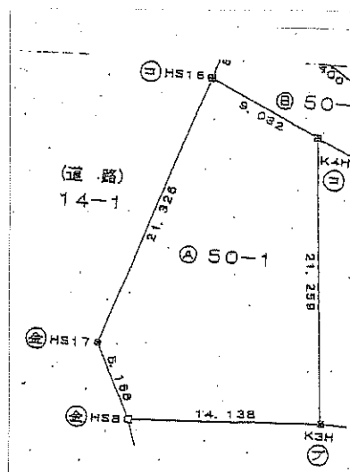
測量図 (1/500)
