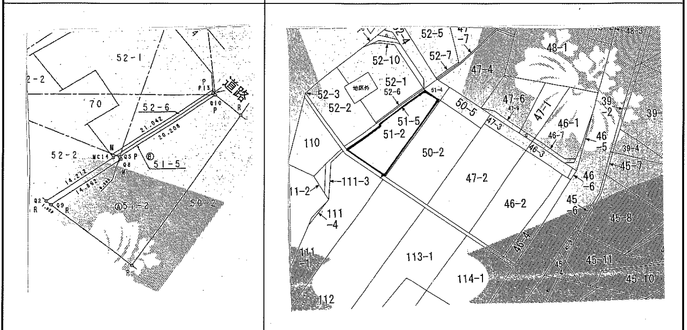
測量図 (1/500を75%縮小) 公図 (1/1000を75%縮小)
