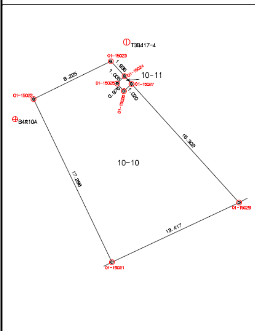
測量図 (1/250を70%縮小)
