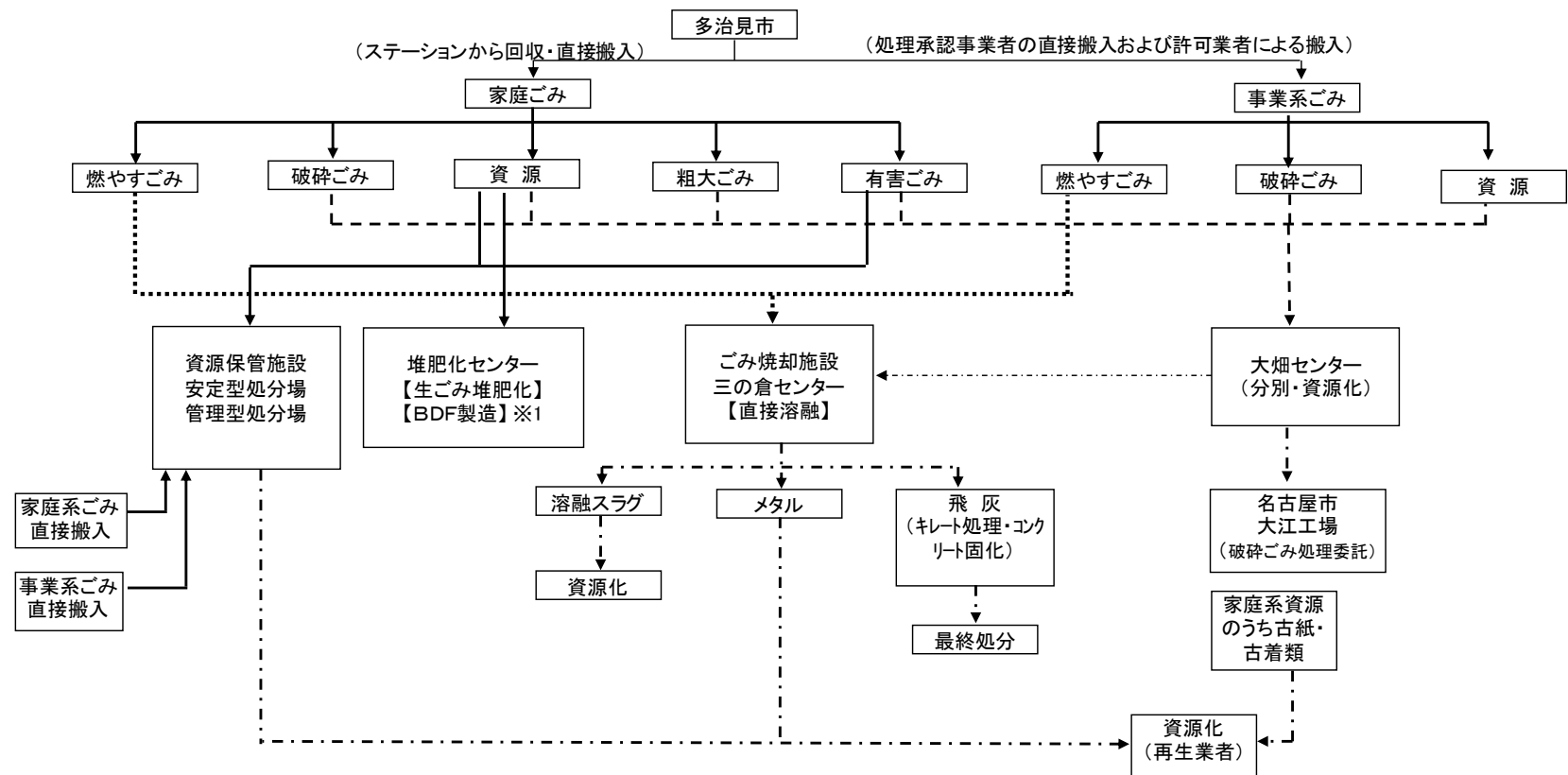
図 3.1 ごみ処理体系
