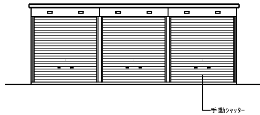
北面 立面図 1/100
