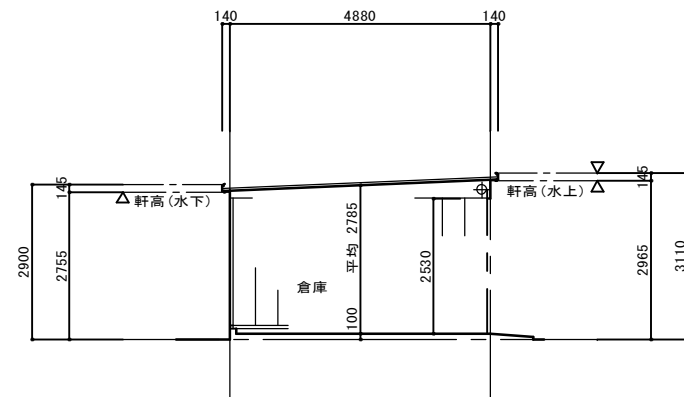
断面図 1/100
