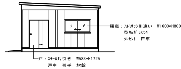
西面 立面図 1/100
