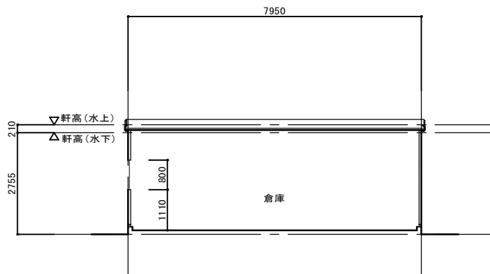
断面図 1/100
