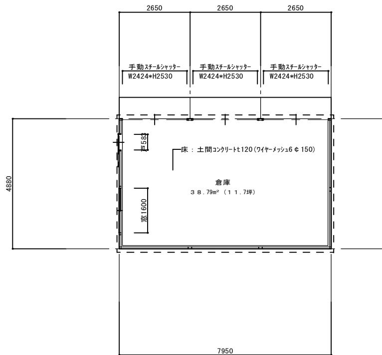
平面図 1/100
