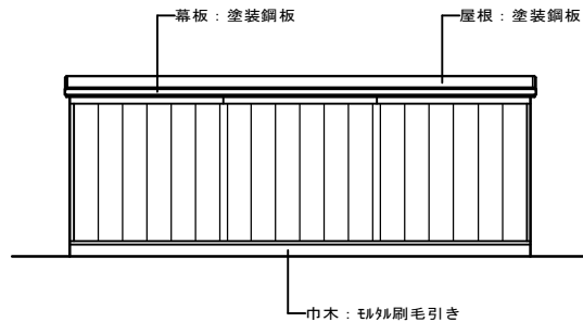
南面 立面図 1/100
