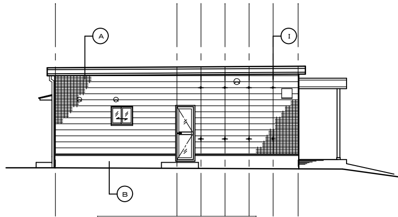
西面 立面図 1/100
