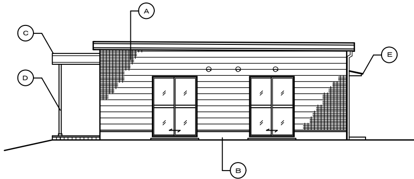
東面 立面図 1/100
