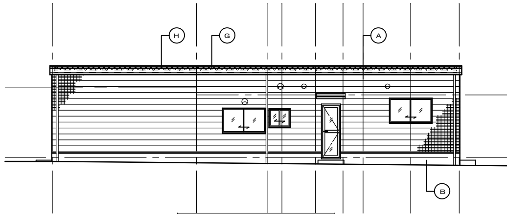
北面 立面図 1/100
