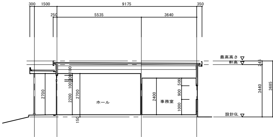
断面図 1/100
