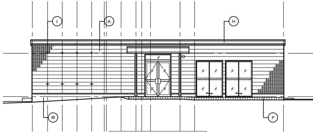
南面 立面図 1/100
