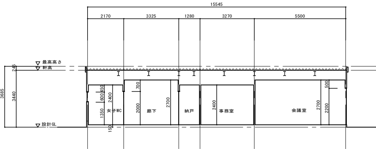
断面図 1/100
