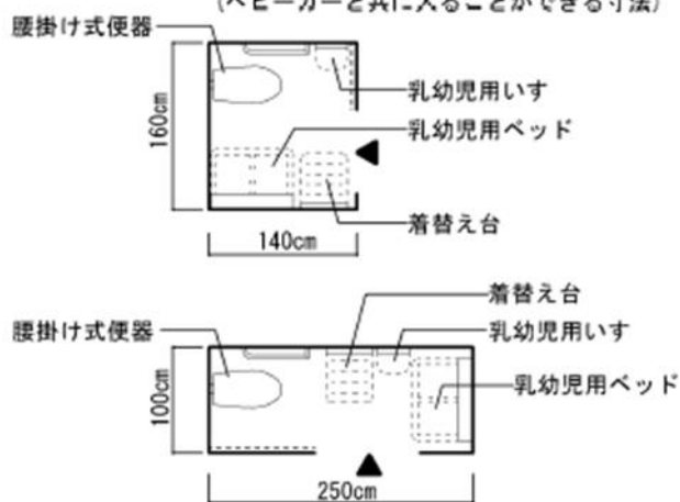
○ 乳幼児連れに配慮した便所の寸法例 (ベビーカーと共に入ることができる寸法)
