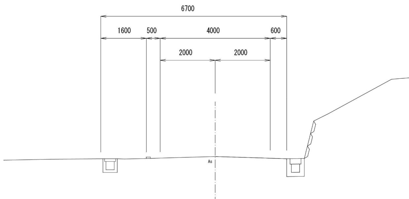
標準断面 (既設断面)
