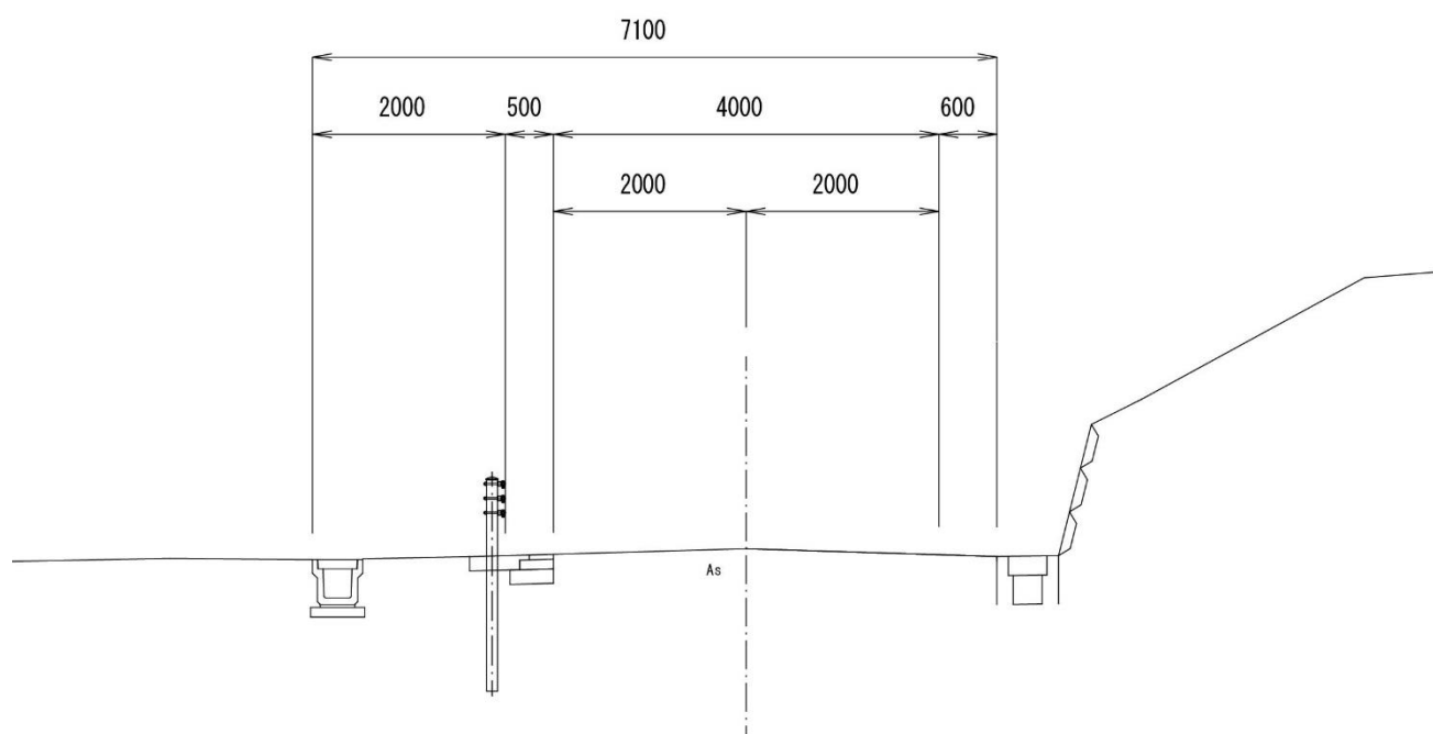
標準断面 (改修後断面)
