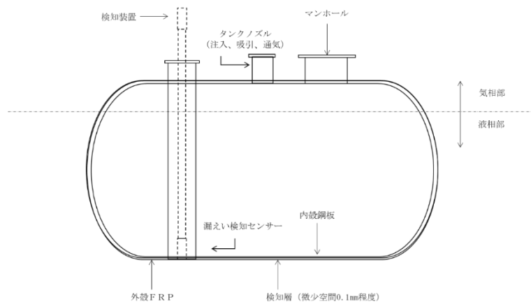
別図1 構造例
