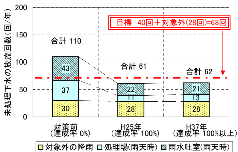
図-7 未処理下水の放流回数（対象外とした降雨を含む場合）
