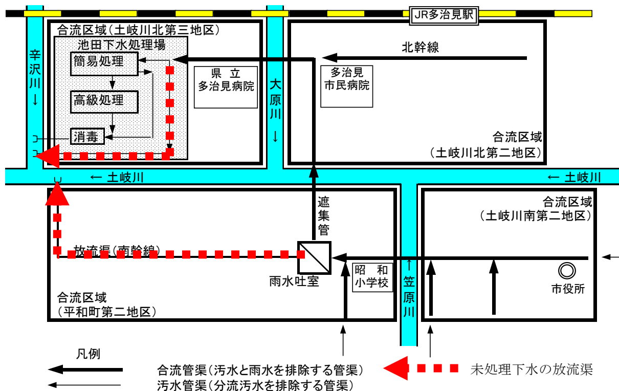
図-2 排水系統模式図
