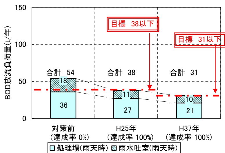
図-5 BOD 年間放流負荷量<<雨天日のみ表示>>
