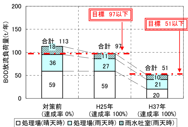
図-4 BOD 年間放流負荷量<<晴天日+雨天日>>
