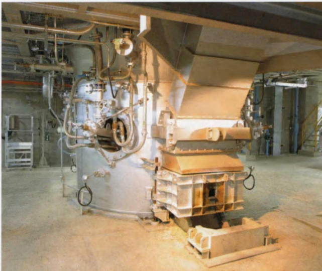
熔融炉（下部）
